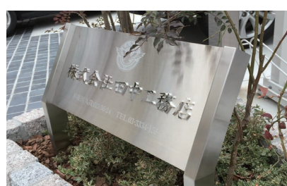
写真 No. 0690-11 切り文字付きステンレス銘板 特注内容：仕様 サイズ：H300×W600mm カラー：文字シルバー、一部切り文字鏡面 納期：デザイン確定後、約 18 日
