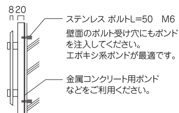
仕様側面図
