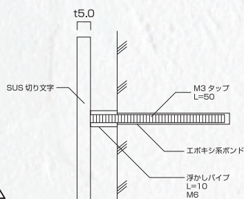
▶側面図
